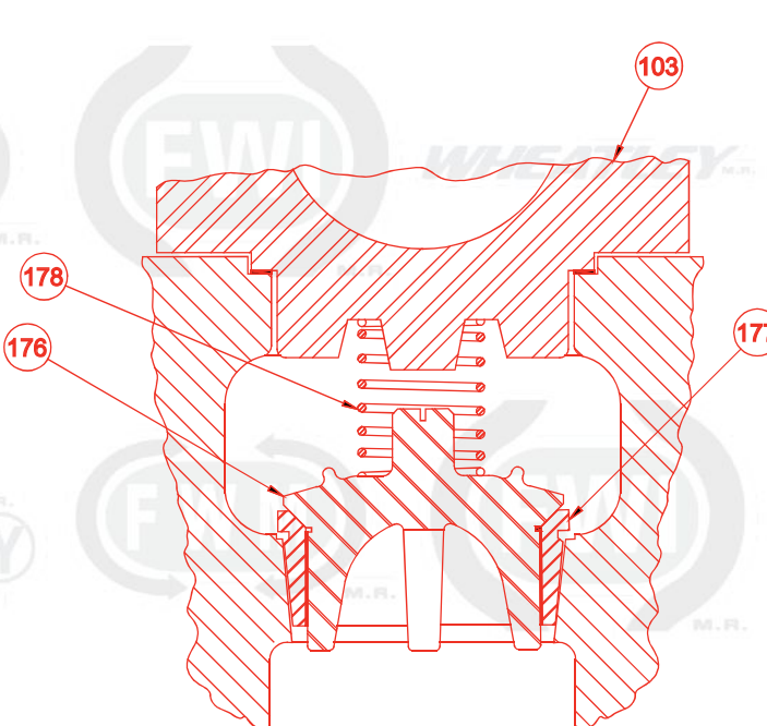
VALVULA ALETA GUIADA DE ACERO TRATADO
