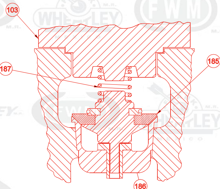
VALVULA SELLO DE HULE
