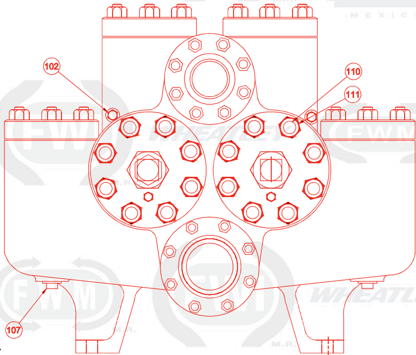
BOMBA DE PISTON DUPLEX FIGURA 6070 LADO FLUIDO 2 1/2 - 5 x 10 1/8
