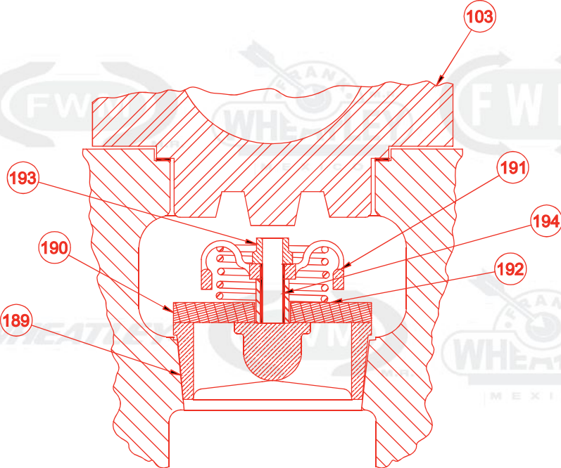
VALVULA DE BRONCE DISCO DE CELCON
