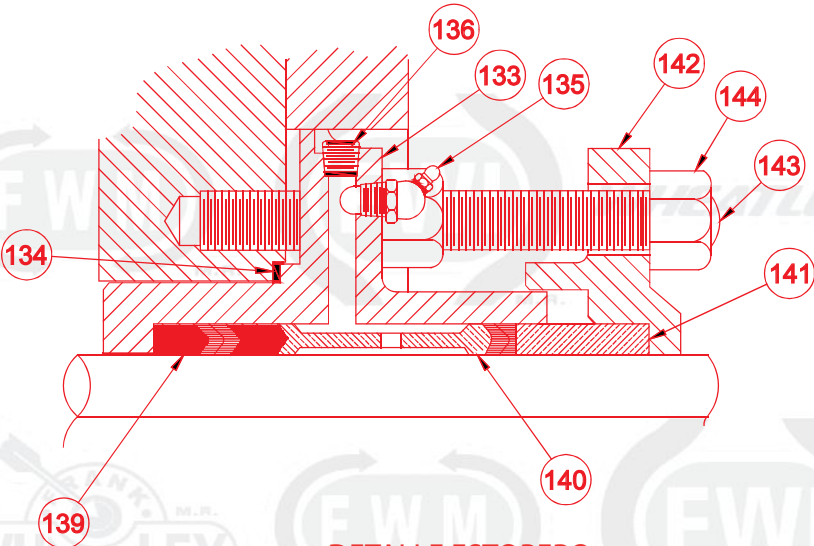
DETALLE ESTOPERO
