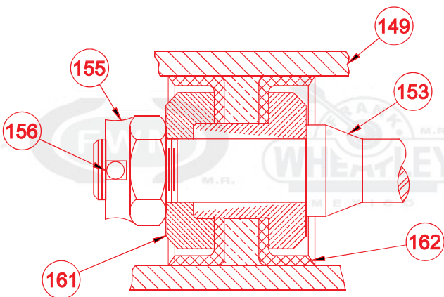
PISTON TIPO COPA
