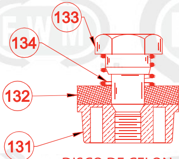
DISCO DE CELON DE VALVULA (BRONCE)
