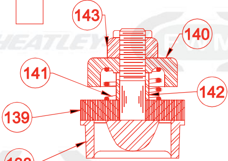
DISCO DE CELCON DE VALVULA (ACERO INOXIDABLE)
