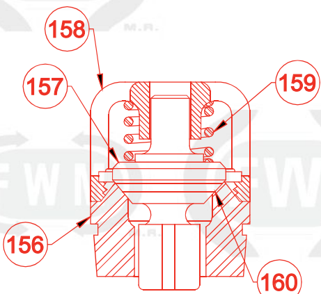
SELLO DE TEFLON DE VALVULA (ACERO & ACERO INOXIDABLE)
